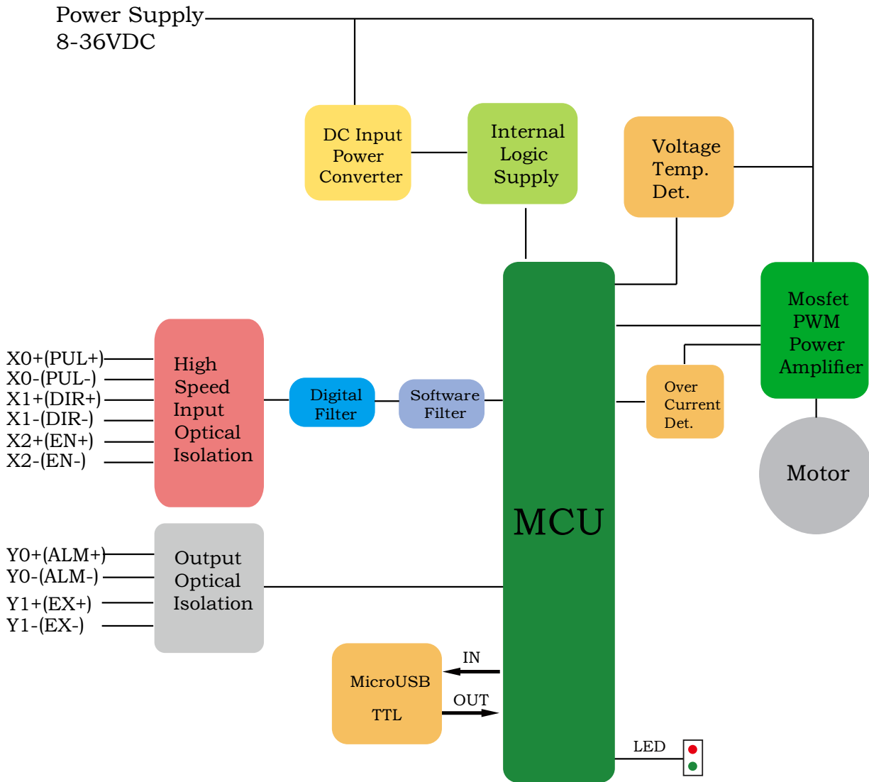
IR35E Block Diagram
